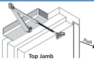
Top Jamb
